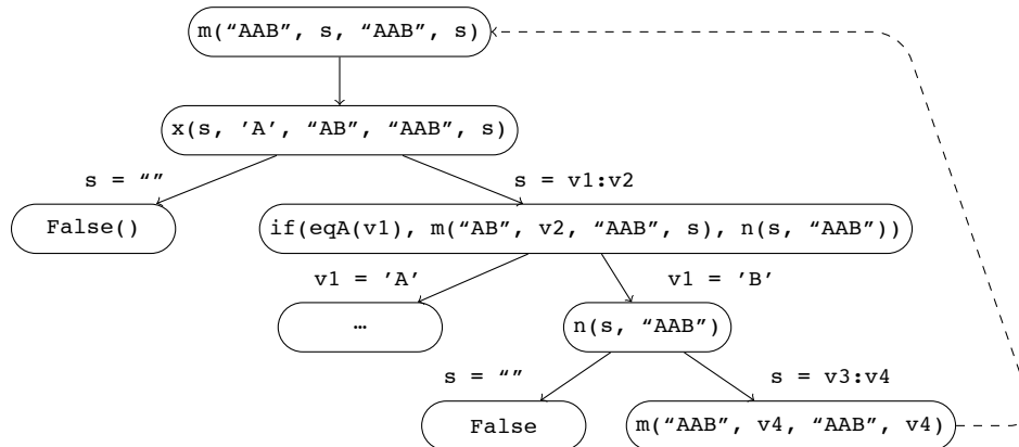
Рис. 7.12. Верхняя часть графа КМПИ-теста после удаления транзитных шагов
