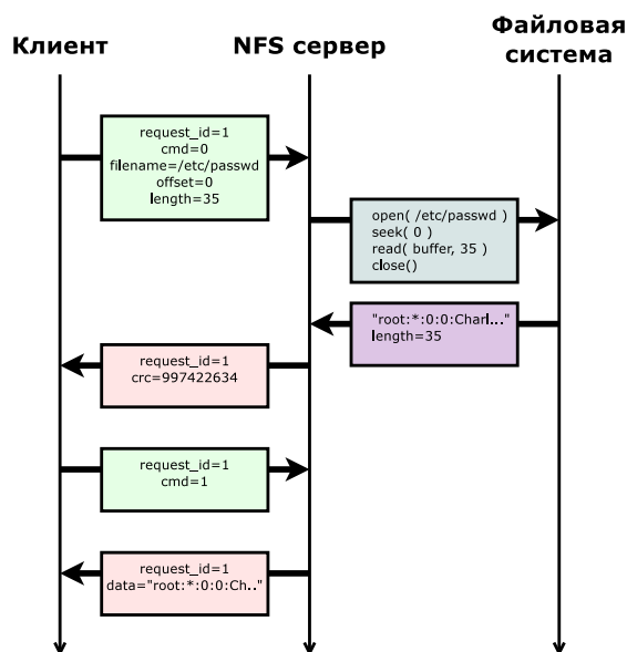
Рис. 6.1. Пример сессии протокола
