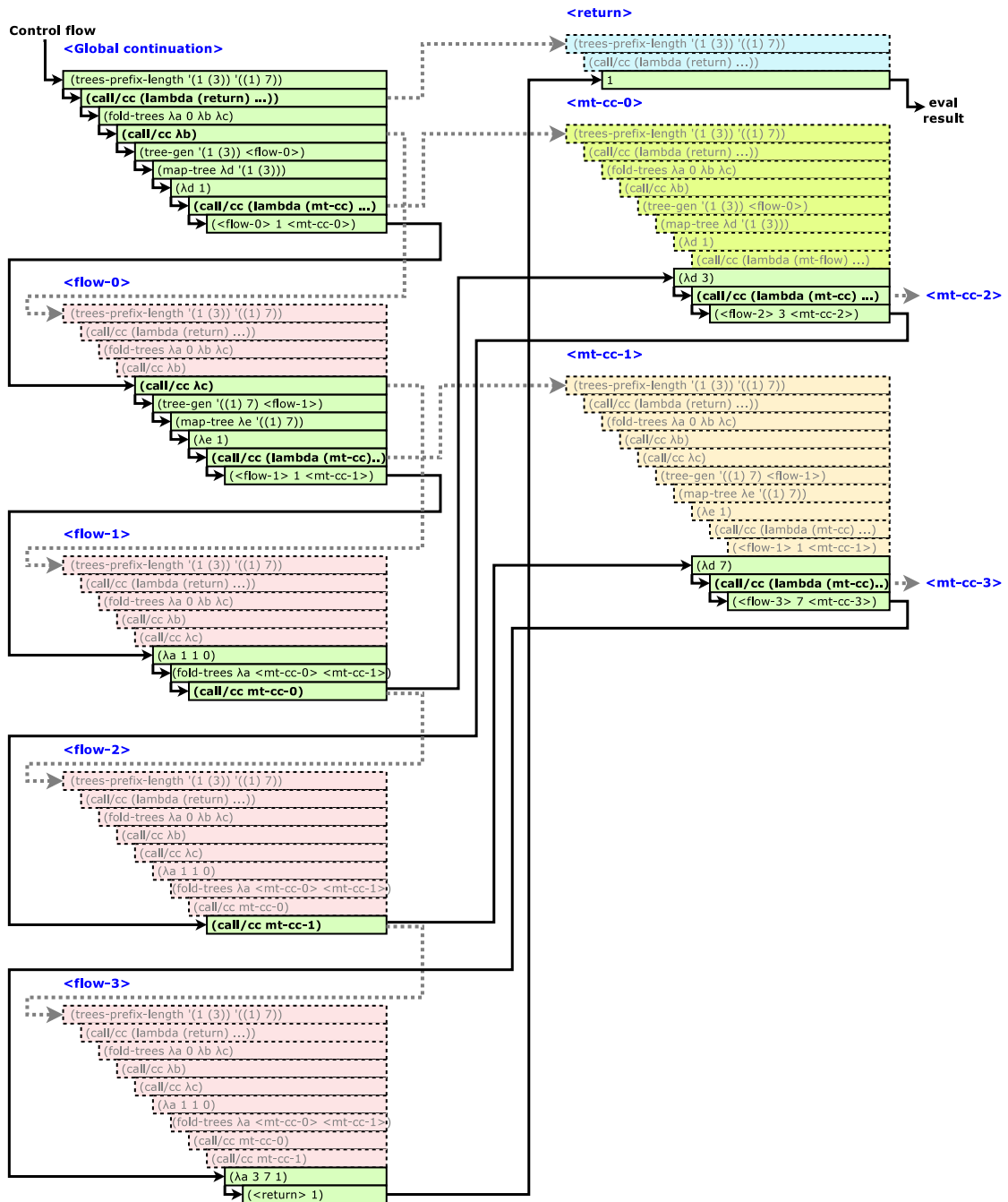
Рис. 6.3. tree-prefix-length, ход выполнения (trees-prefix-length '(1 (3)) '((1) 7))
