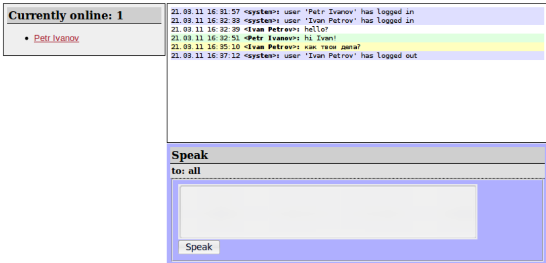
Рис. 6.7. weblocks-chat
