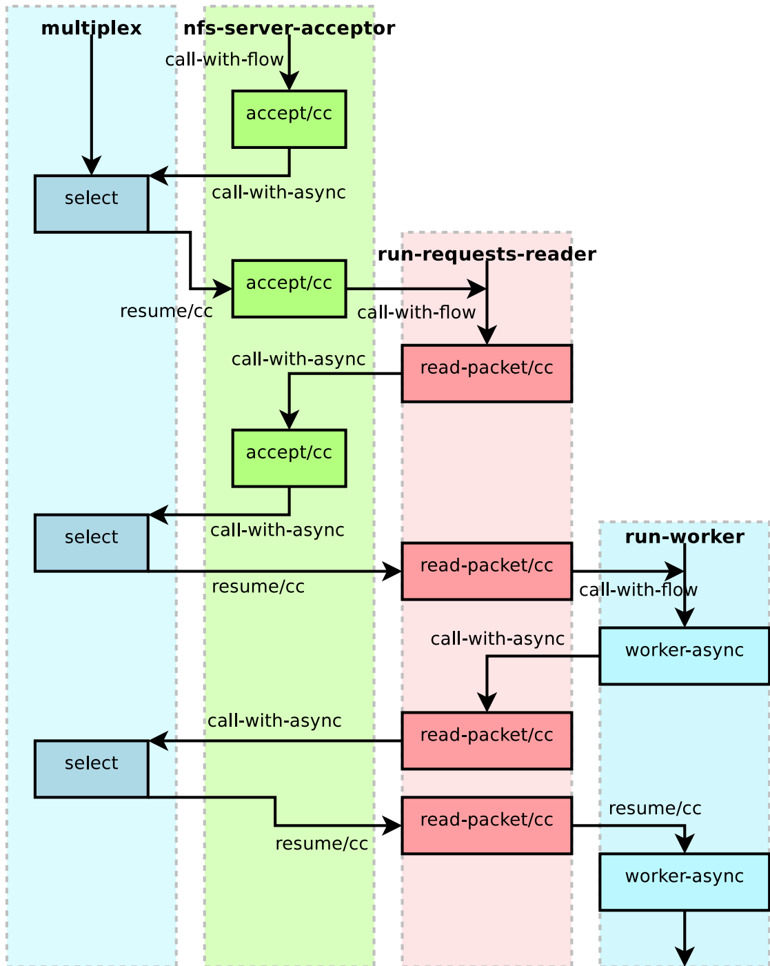
Рис. 6.4. Ход выполнения программы
