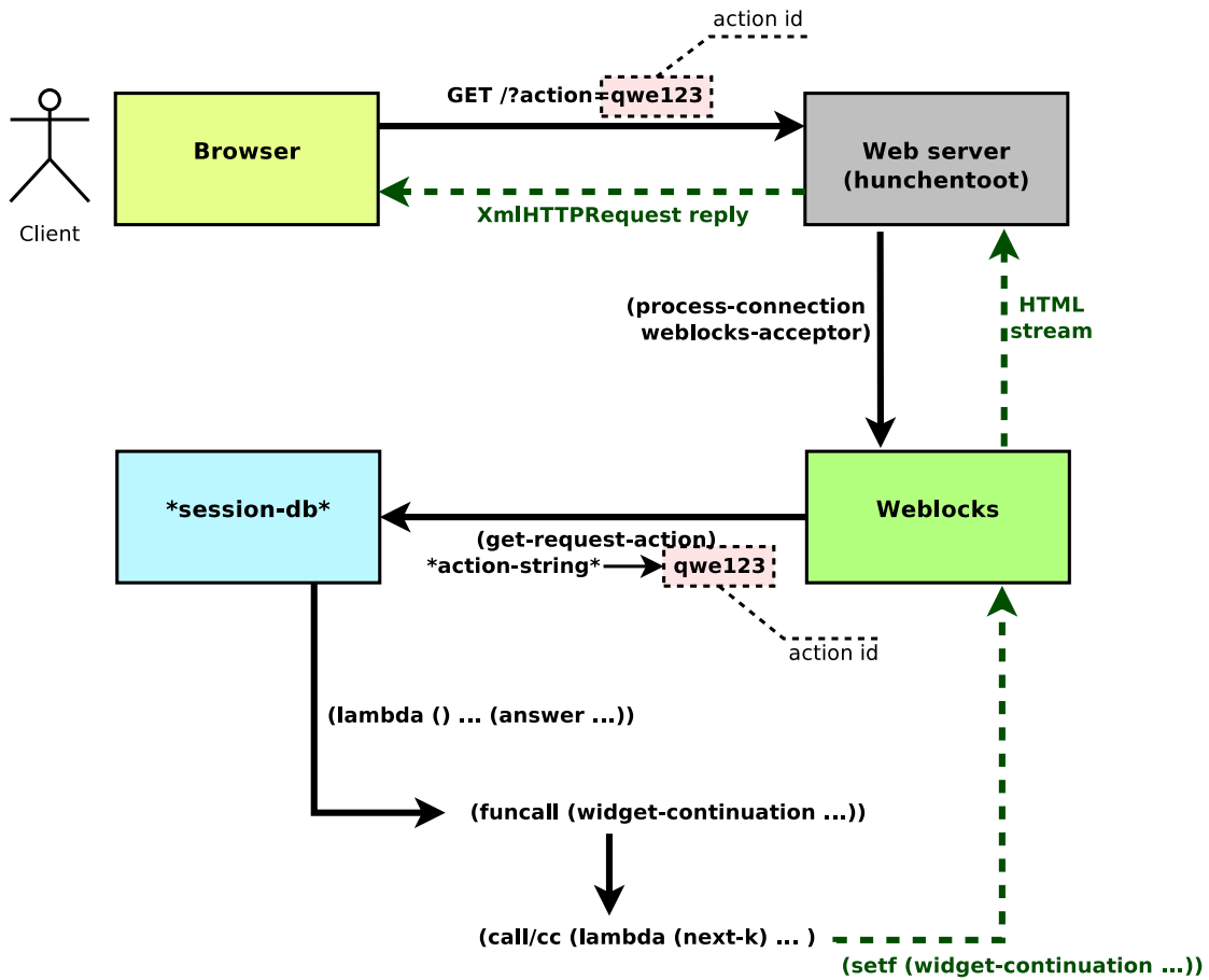
Рис. 6.5. Передача управления при HTTP запросе в Weblocks
