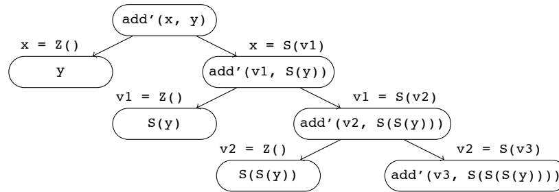
Рис. 7.8. Дерево конфигураций для задания (\text{add}'(x, y), \text{prog1})
