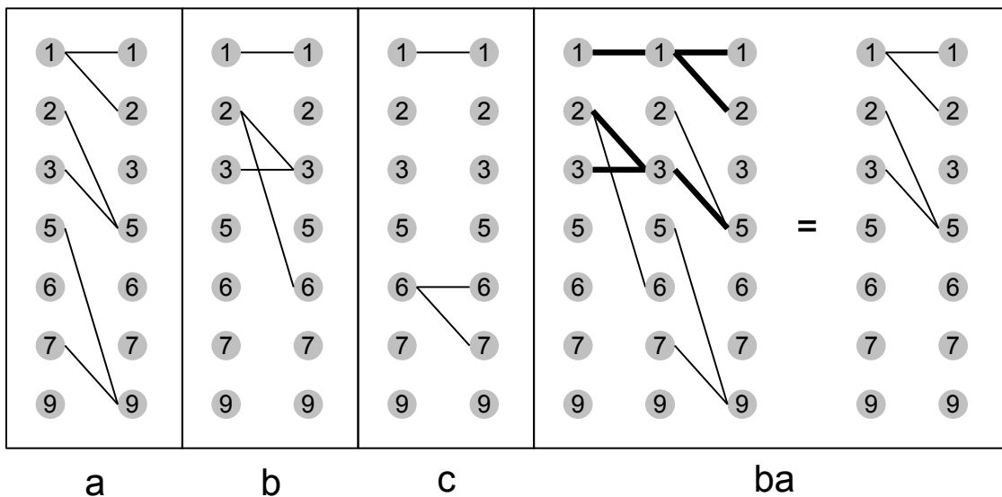
Рис. 6.4. Переходные функции недетерминированного автомата и их композиция
