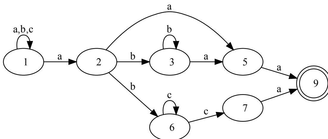
Рис. 6.2. Недетерминированный автомат, соответствующий выражению « \cdot * a (b * a | bc + ) a », после удаления \epsilon -дуг
