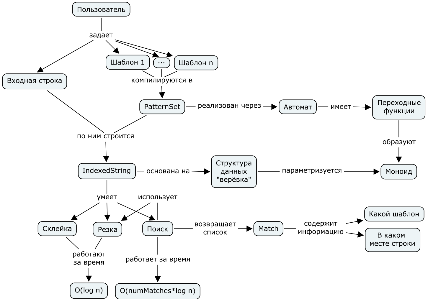
Рис. 6.9. Общая схема программы
