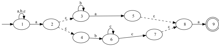
Рис. 6.1. Недетерминированный автомат, соответствующий выражению «. *a (b*a | bc+) a»
