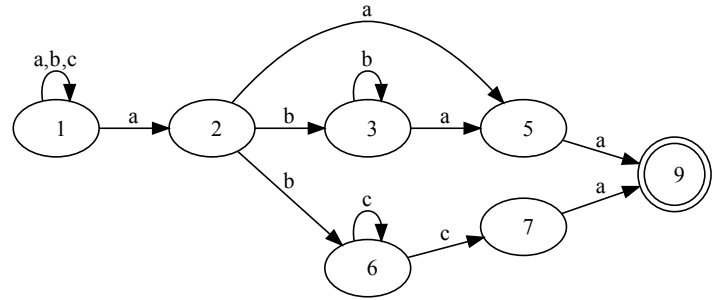
Рис. 6.2. Недетерминированный автомат, соответствующий выражению «. *a (b*a | bc+) a», после удаления \epsilon -дуг
