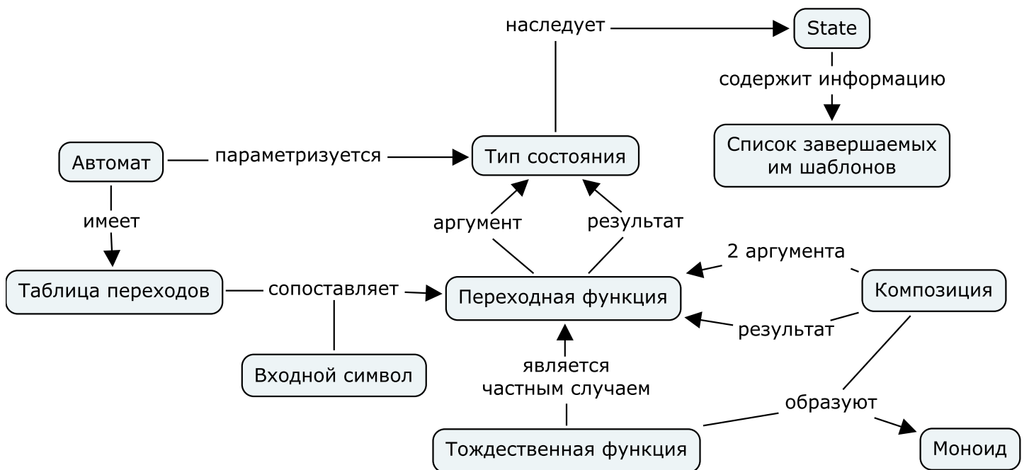
Рис. 6.11. Схема программы: Конечные автоматы
