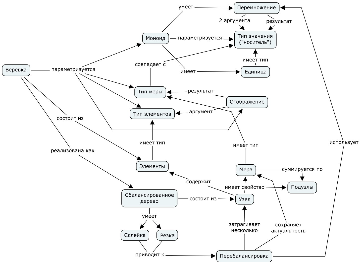
Рис. 6.10. Схема программы: Верёвки и моноиды
