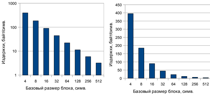
Рис. 6.16. Издержки потребления памяти
