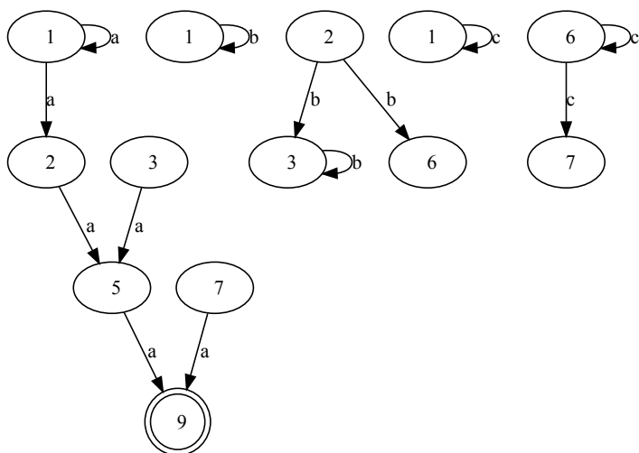
Рис. 6.3. Недетерминированный автомат, соответствующий выражению « \cdot * a (b^* | c^+) a », расслóнный посимвольно
