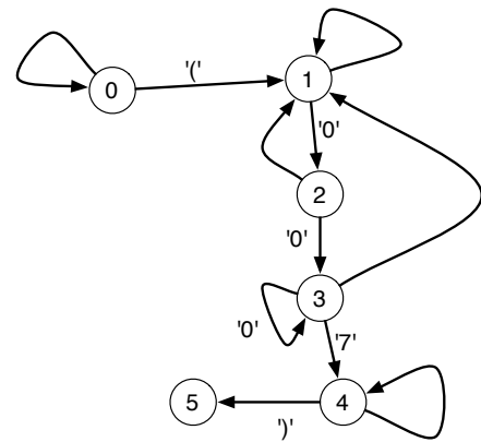
Рис. 5.1. Автомат для выражения .*(.*007.*).*
