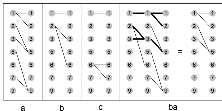
Рис. 6.4. Переходные функции недетерминированного автомата и их композиция
