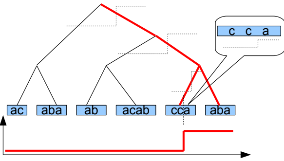
Рис. 6.6. Разрезание верёвки для строки acabaabacabssaaba по монотонному условию «содержит bcc »
