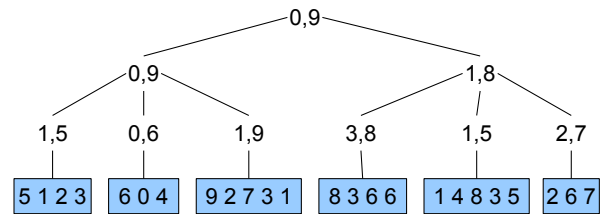
Рис. 6.8. Пример верёвки из чисел с заэкшированным минимумом и максимумом
