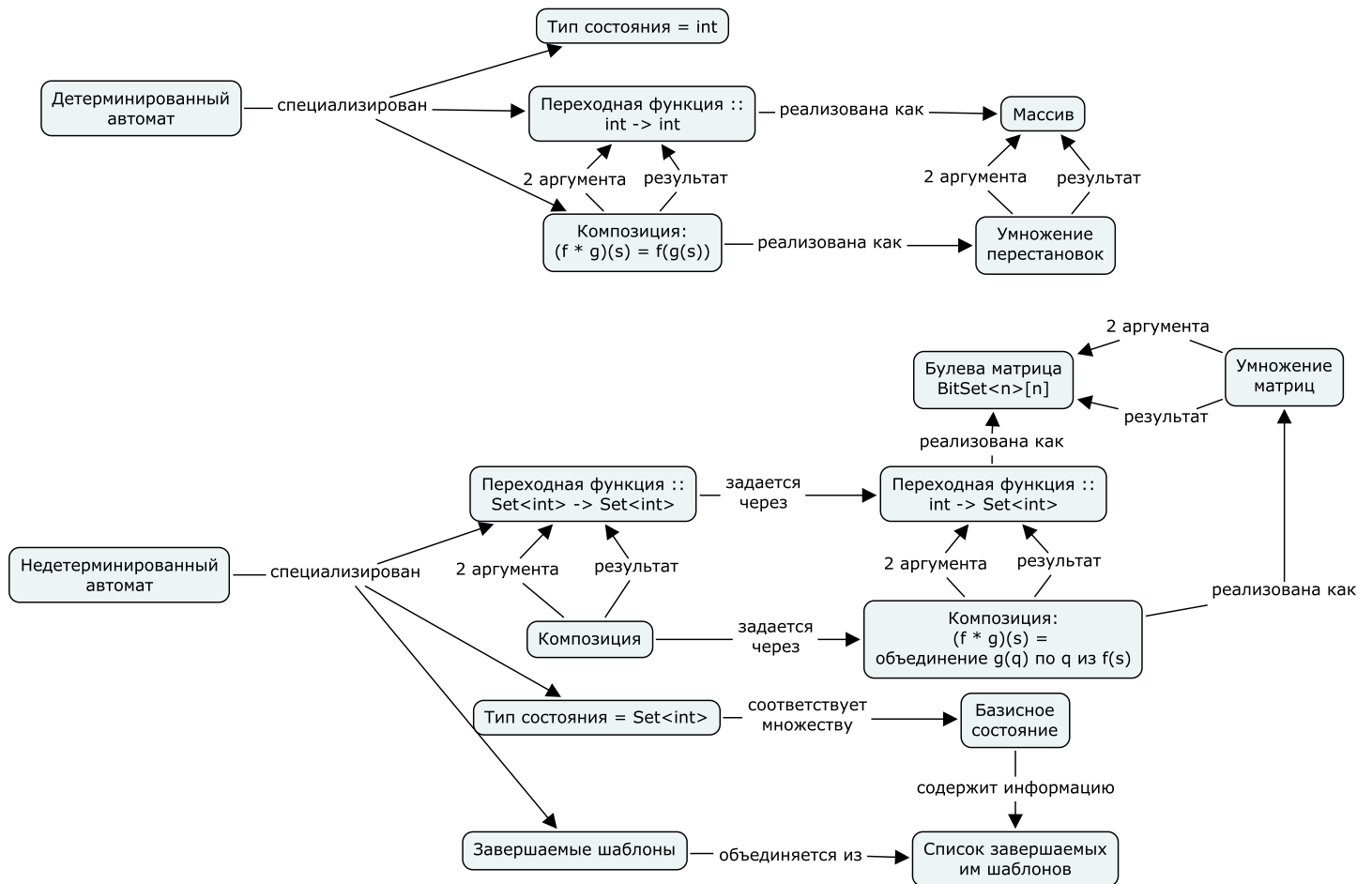
Рис. 6.12. Схема программы: Связь детерминированных и недетерминированных автоматов
