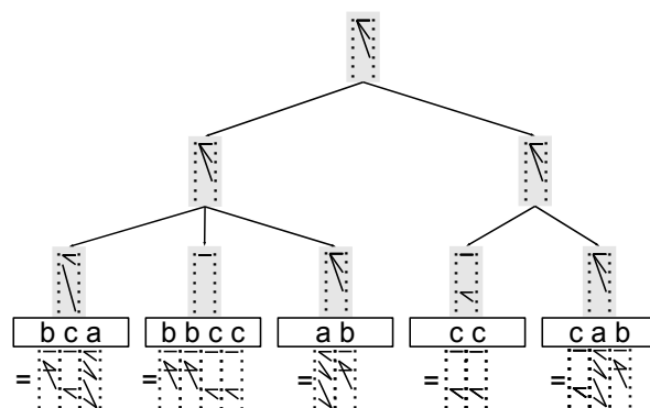
Рис. 6.5. Пример верёвки с закэшированной переходной функцией относительно выражения « \cdot * a (b^* | c^+) a » для строки bcabbccabcccab
