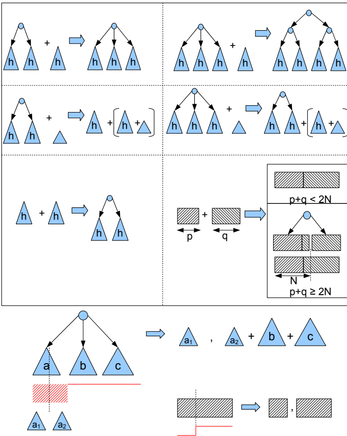
Рис. 6.13. Операции над веревками
