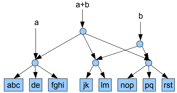
Рис. 6.14. Совместное использование памяти при склейке верёвок
