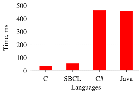
Рис. 1.3. Программистский супертест, без Erlang
