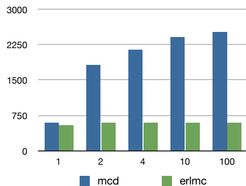
Рис. 2.5. Сравнение скорости mcd и erlmc на 10 килобайтах данных
