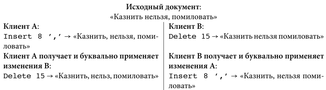
Рис. 3.1. Конфликты, возникающие при наивном подходе к объединению правок
