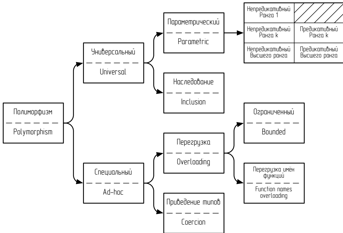
Рис. 4.1. Классификация видов полиморфизма в языках программирования
