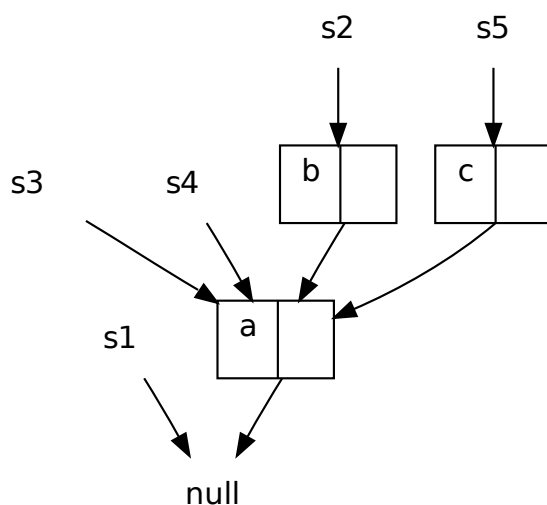
Рис. 5.3. Диаграмма объектов к коду примера со стеками
