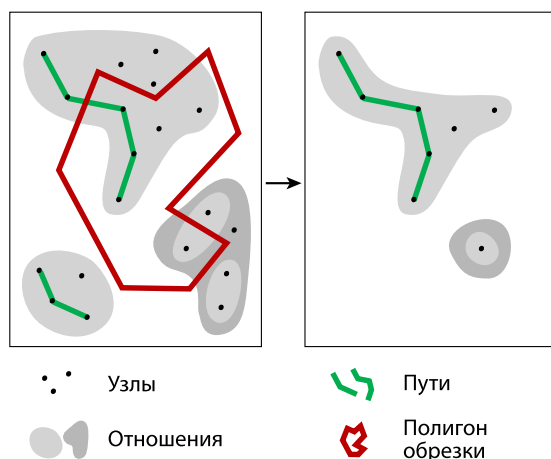
Рис. 1. Пример фильтрации с опцией completeObjects
