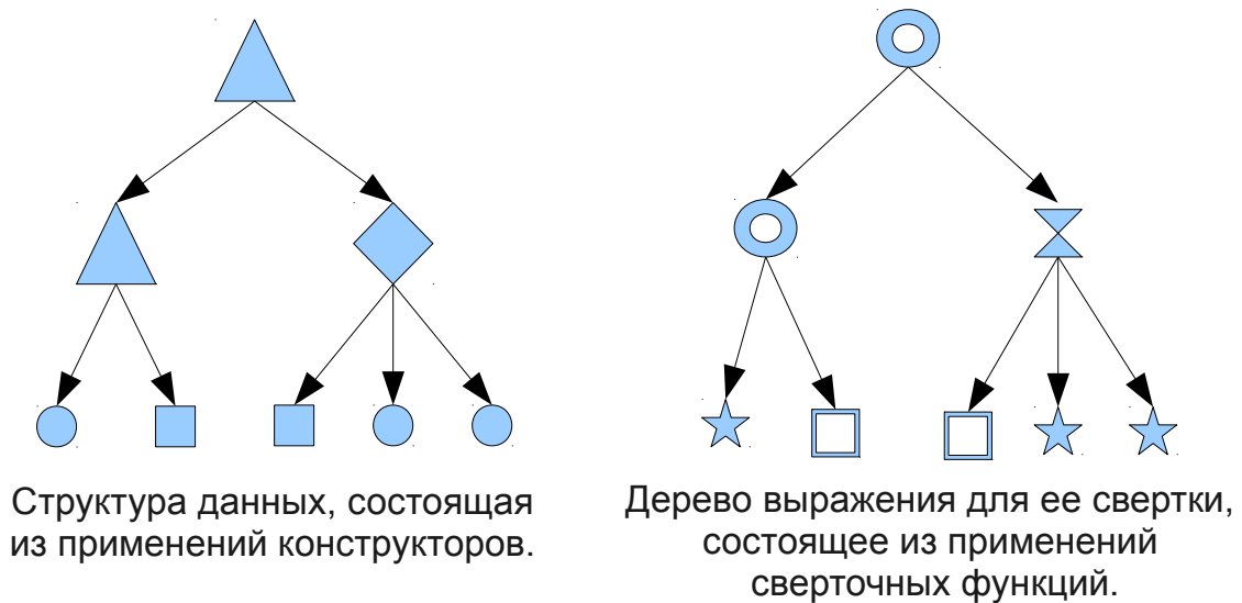
Рис. 5.7. Свёртка как подмена конструкторов
