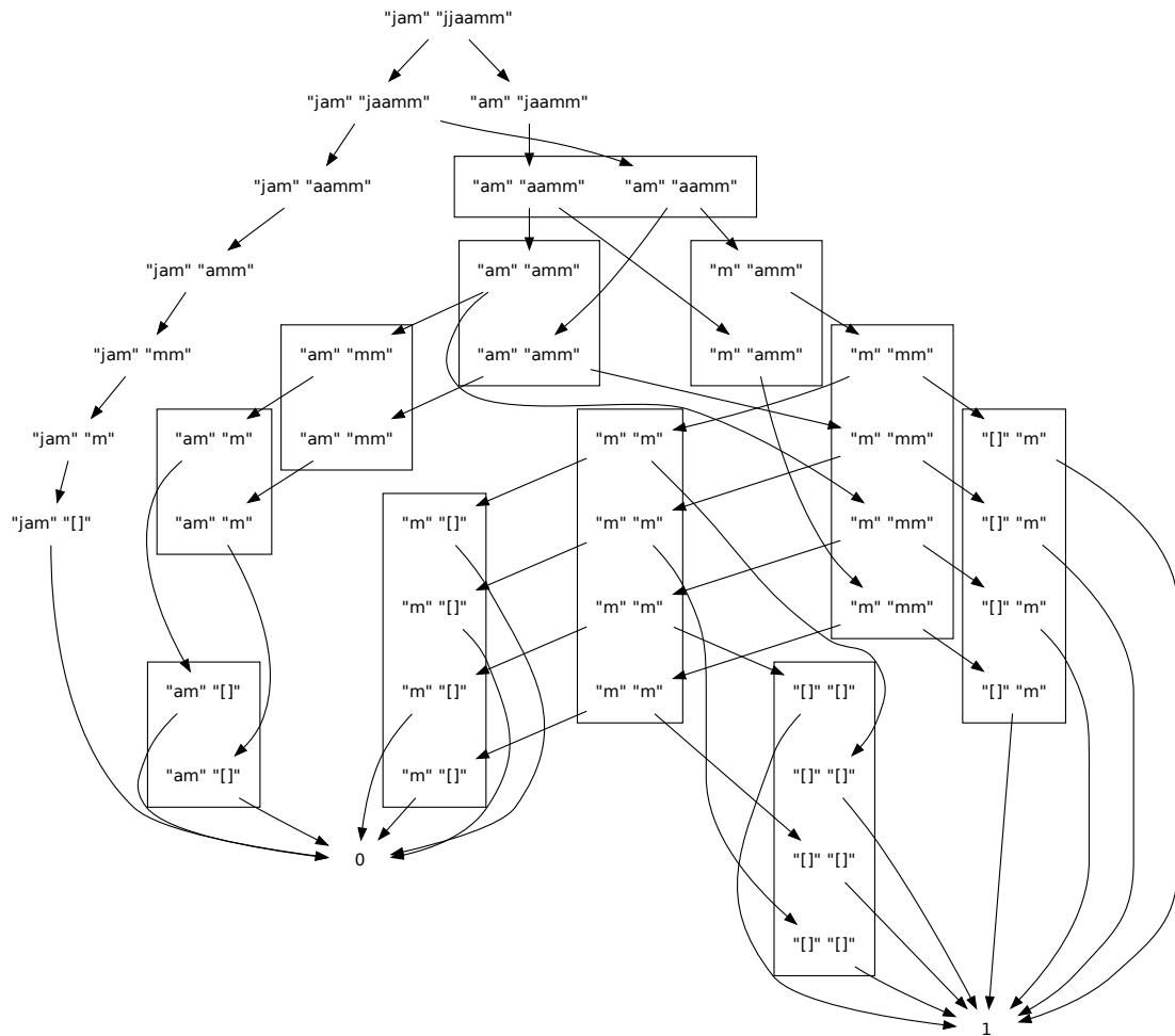
Рис. 1.1. Вычисление occurs "jam" "jjaamm"
