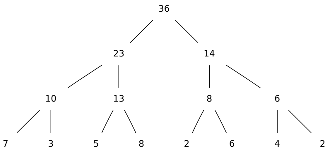
Рис. 5.8. Дерево вычисления ассоциативной свертки по сложению
