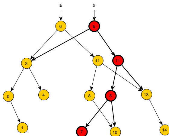
Рис. 5.4. Чисто функциональные деревья
