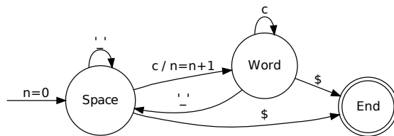
Рис. 5.2. Конечный автомат для подсчета слов
