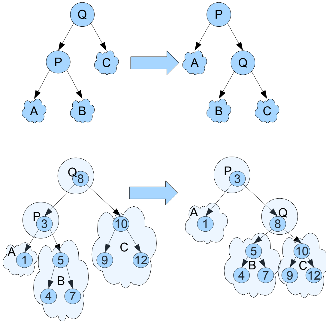
Рис. 5.6. Правый поворот дерева
