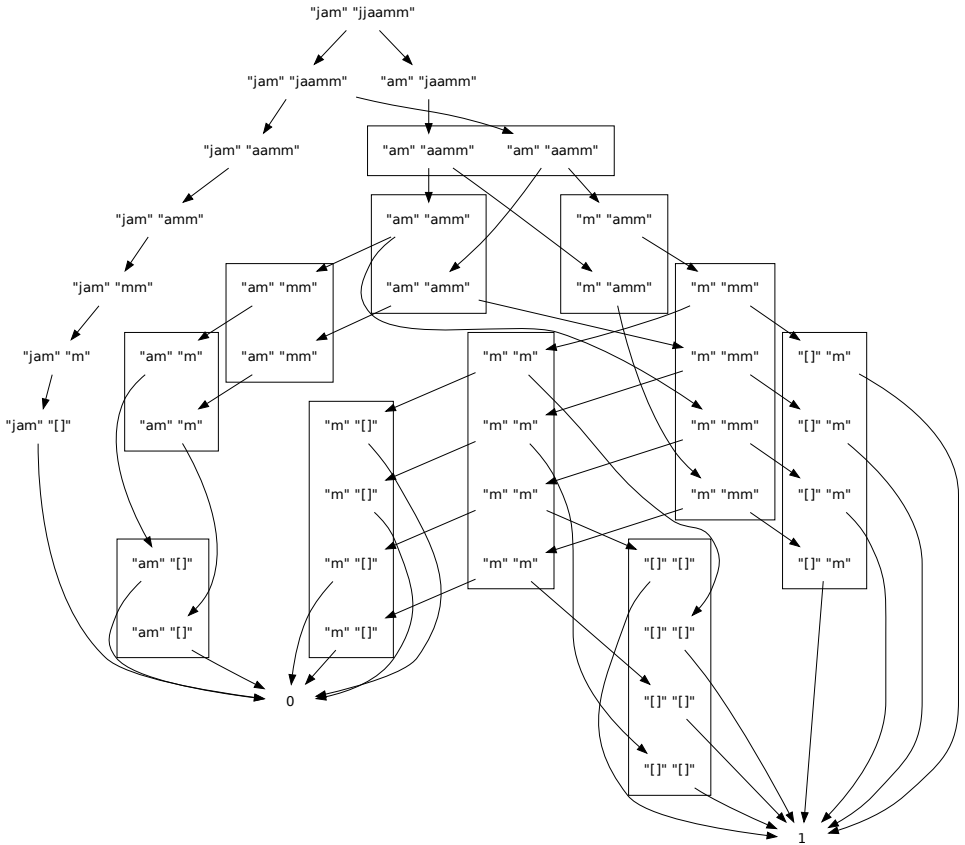
Рис. 1.1. Вычисление occurs "jam" "jjaamm"
