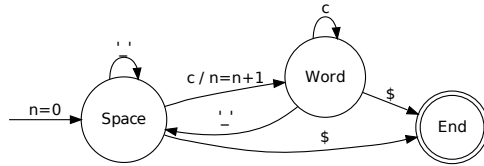
Рис. 5.2. Конечный автомат для подсчета слов
