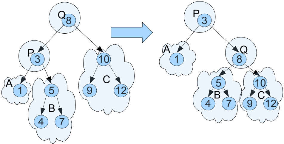
Рис. 5.6. Правый поворот дерева
