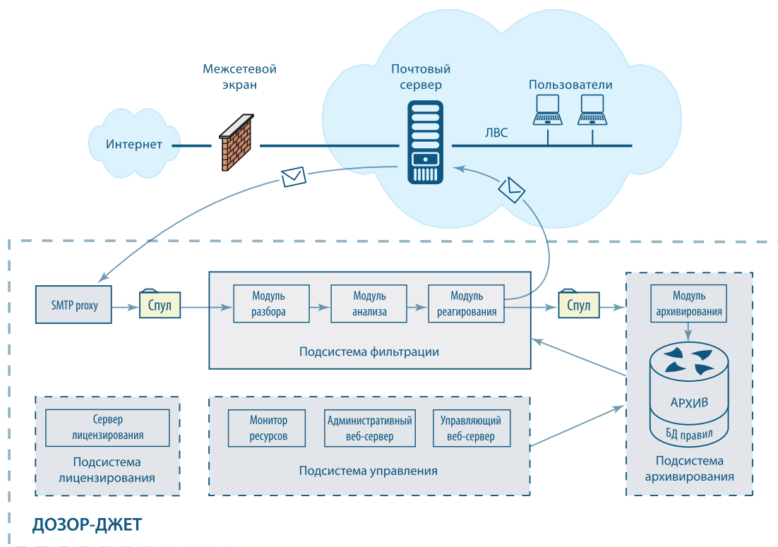
Рис. 4.1. Архитектура СМАП «Дозор-Джет»
