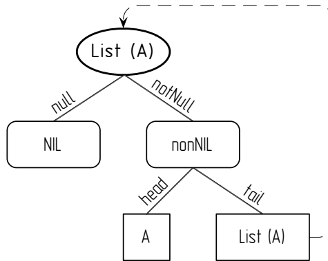
Рис. 6.3. Древоподобное представление типа List(A)
