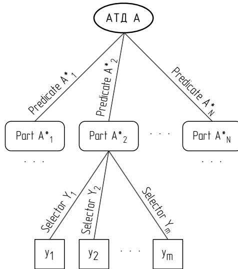
Рис. 6.2. Древоподобное представление АТД
