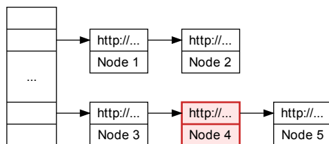
Рис. 3.1. Организация объекта класса HashMap
