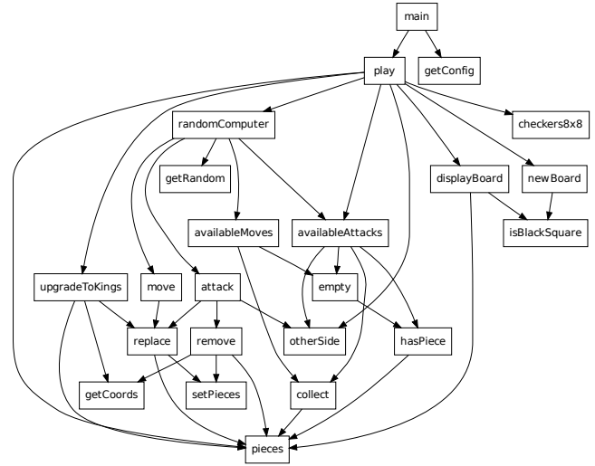
Рис. 4.4. Дерево вызовов функций программы checkers12.hs
