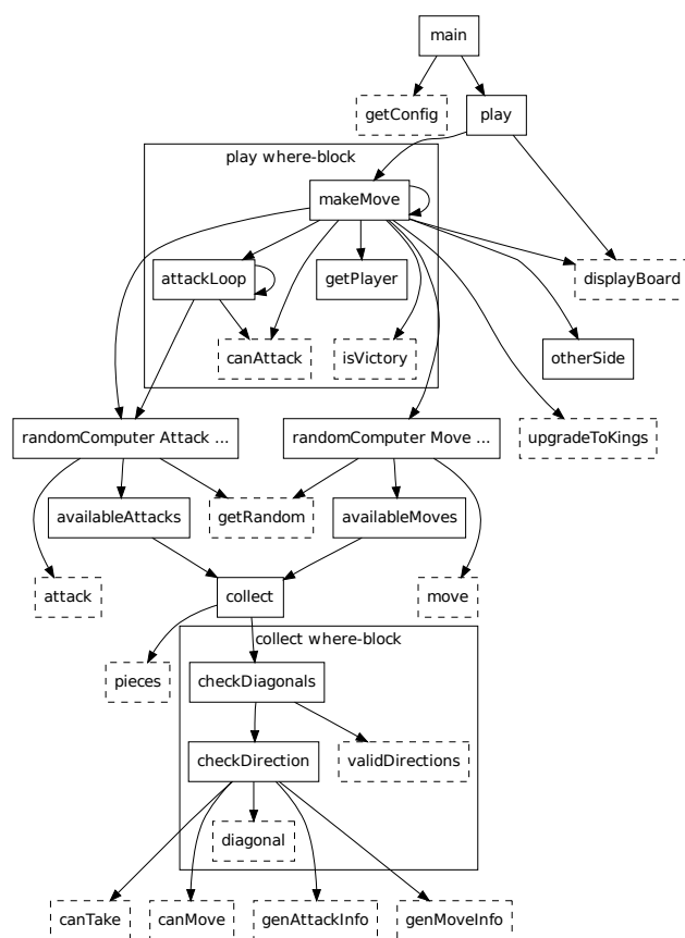
Рис. 4.2. Дерево вызовов функций в файле checkers04.hs
