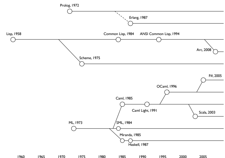
Рис. 6.1. Генеалогическое дерево семейств функциональных и декларативных языков
